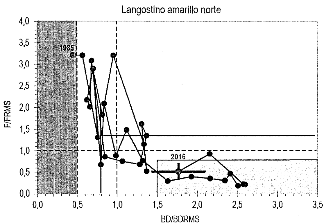
Figura 1: Diagrama de fase del langostino amarillo, área norte
